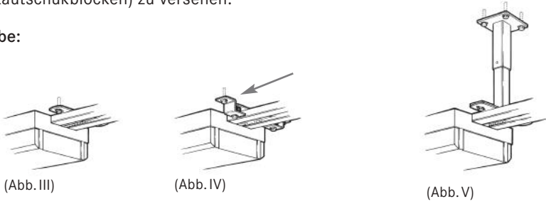
Abb. III: Deckenmontage direkt Abb. IV: Deckenmontage mit vibrationsisolierender Deckenaufhängung Abb. V: Deckenmontage herabgesetzt mit Teleskop-Deckenkonsole (bis 2000mm)
